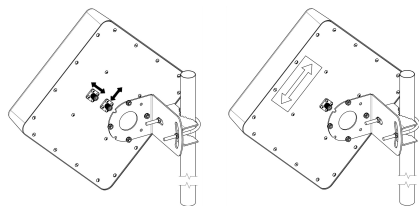
Рисунок 3 – X-поляризация
