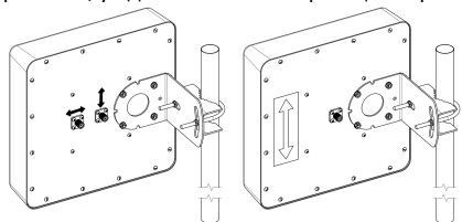
Рисунок 2 – Монтаж антенны на мачте
