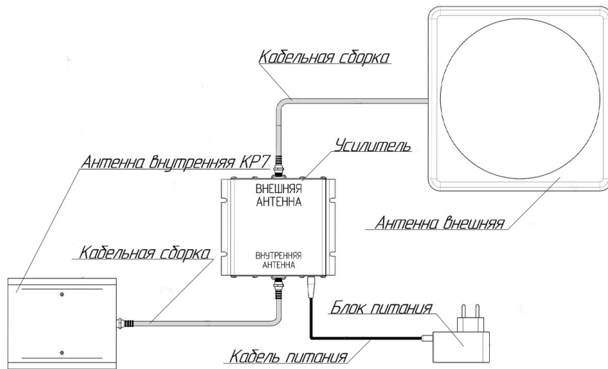
Схема подключения антенны KP7 в системе усиления мобильного сигнала
