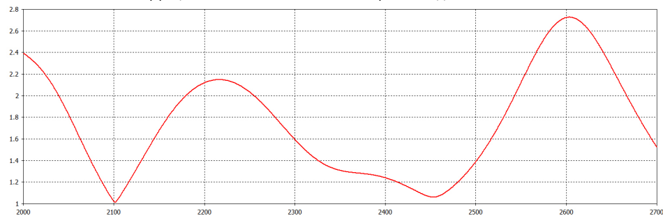
Коэффициент стоячей волны антенны в рабочем диапазоне частот
