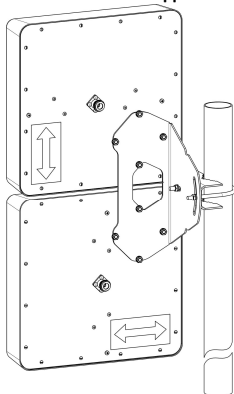
Рисунок 2 – Монтаж антенны на мачте
