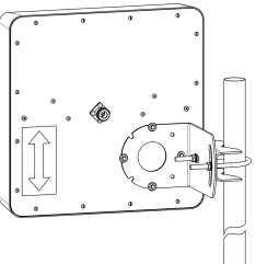
Рисунок 3 – Монтаж антенны на мачте
