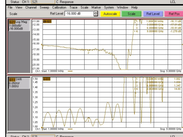
Графики для АЧХ - Log Mag, при отсчётном уровне равном -16 дБ, и для КСВ - SWR
