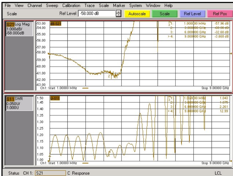
Графики для АЧХ - Log Mag, при отсчётном уровне равном -58 дБ, и для КСВ – SWR
