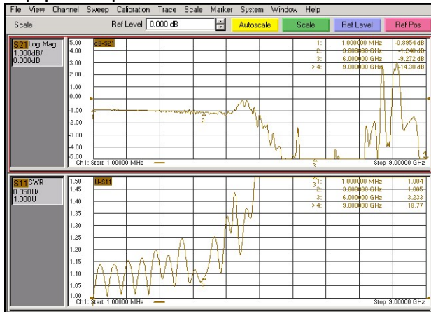
Графики для АЧХ - Log Mag, при отсчётном уровне равном 0 дБ, и для КСВ - SWR
