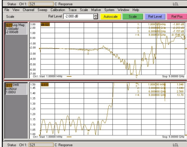
Графики для АЧХ - Log Mag, при отсчётном уровне равном -2 дБ, и для КСВ - SWR
