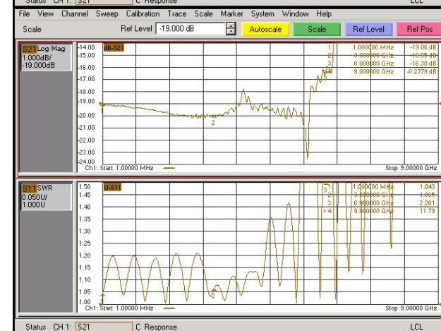
Графики для АЧХ - Log Mag, при отсчётном уровне равном -19 дБ, и для КСВ - SWR
