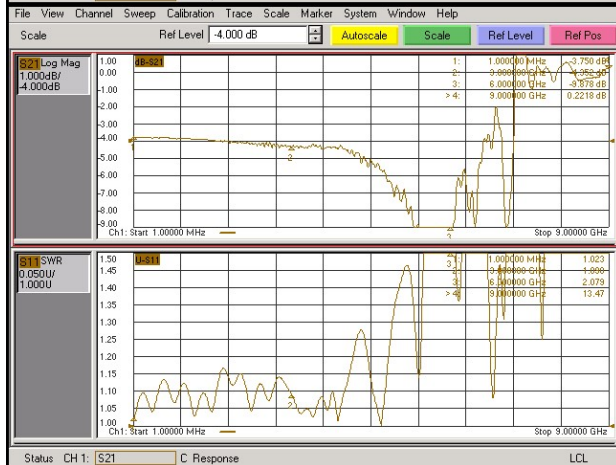
Графики для АЧХ - Log Mag, при отсчётном уровне равном -4 дБ, и для КСВ - SWR
