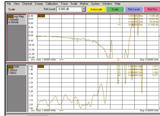
Графики для АЧХ - Log Mag, при отсчётном уровне равном -8 дБ, и для КСВ - SWR
